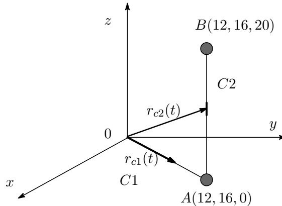
図 2: 積分経路
