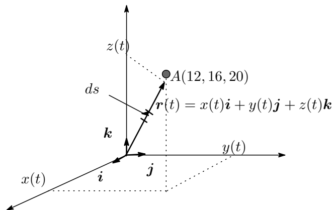
図 1: 積分経路
